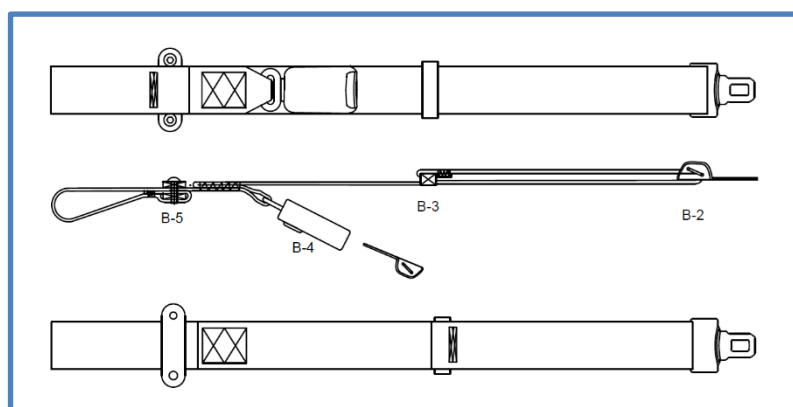
Sistema de cierre con Hebilla y Lengüeta
